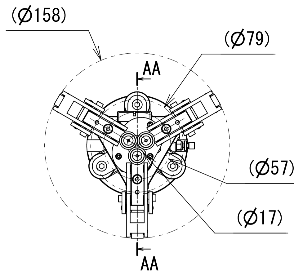
3等配閉寸法
