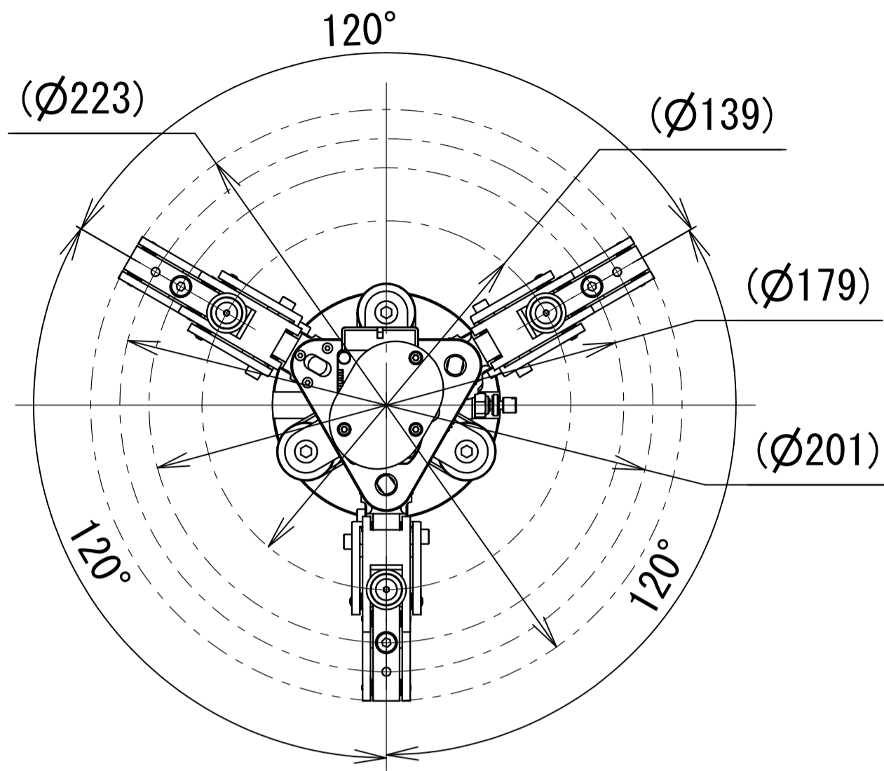
3等配開寸法
