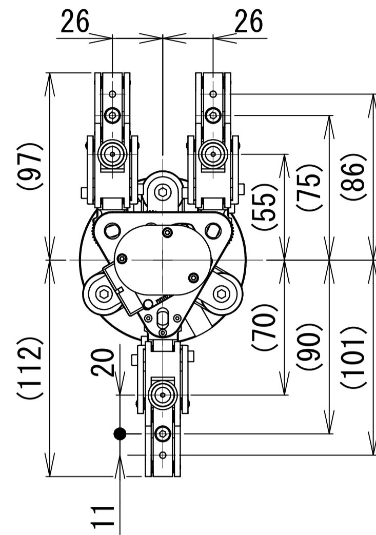
対向開寸法
