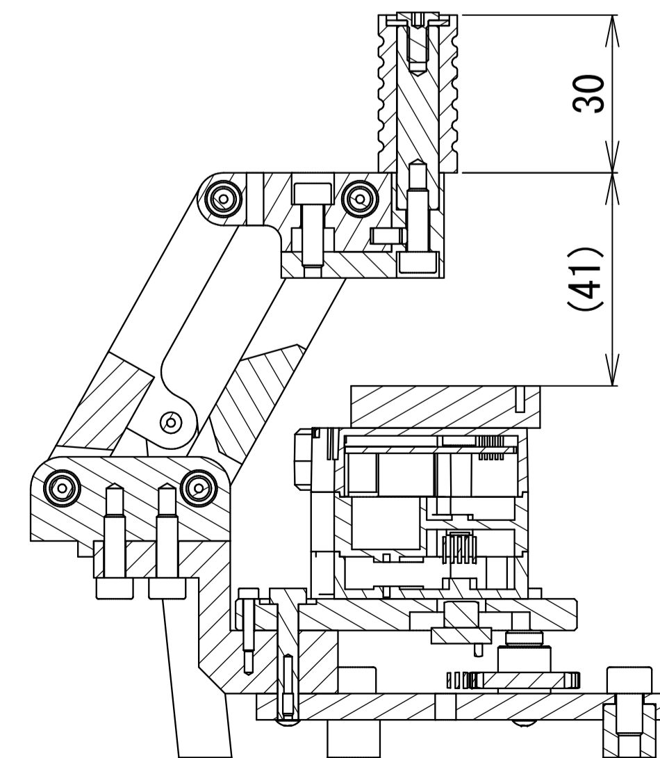
AB-AB (1:1)
